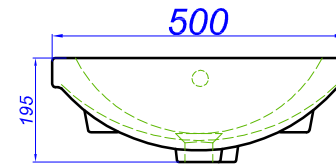
Вид спереди
